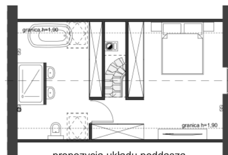
propozycja układu poddasza
